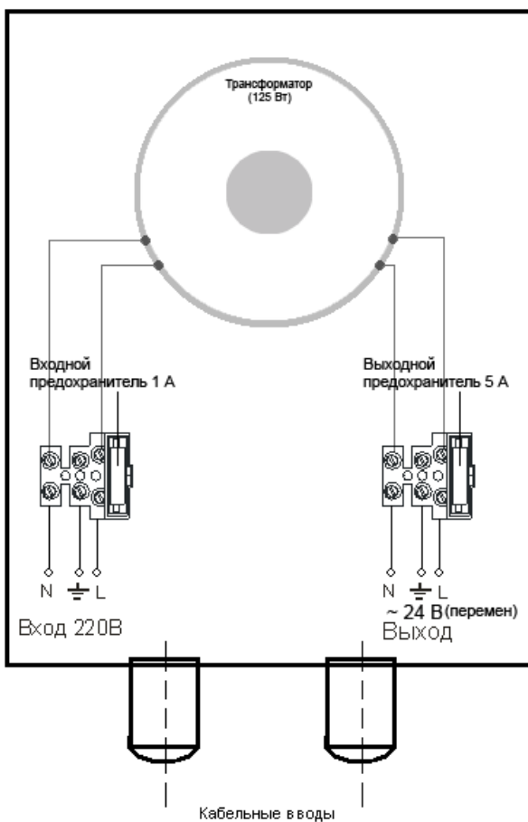
Схема подключения источника согласно рис. 1
