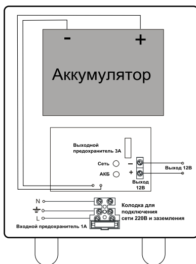
Схема подключения источника согласно рис. 1
