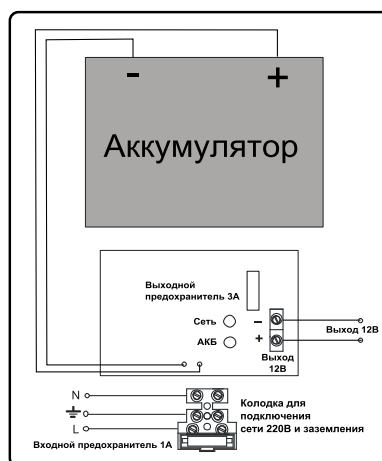
Схема подключения источника согласно рис. 1
