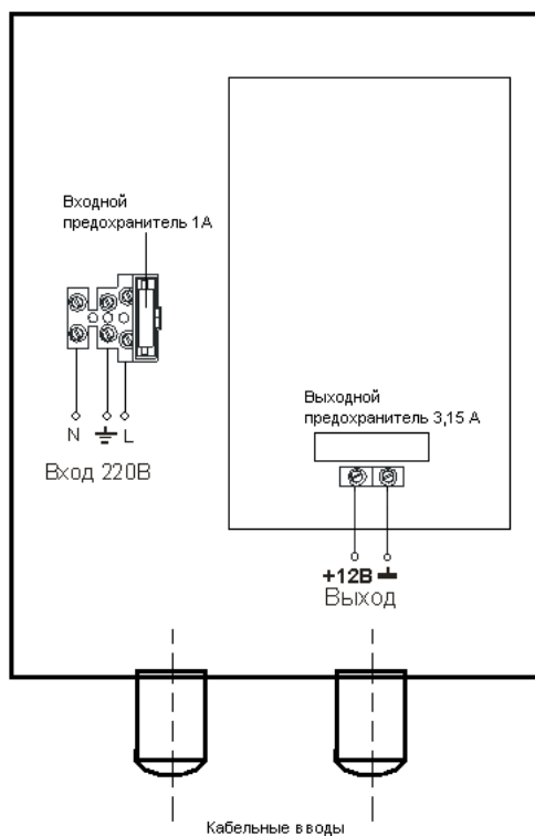
Схема подключения источника согласно рис. 1
