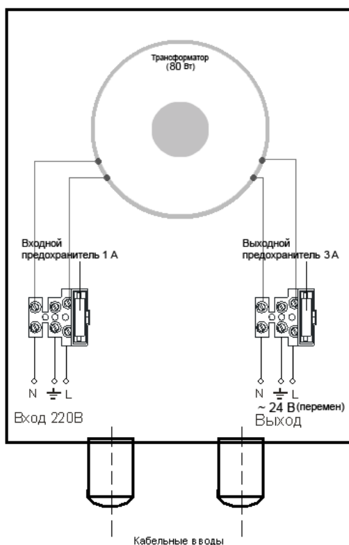
Схема подключения источника согласно рис. 1
